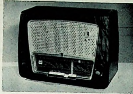
BX 533 A f 348,- afm. 38 x 52 x 24 cm vier golfgebieden, incl. F.M.-band 9 buizen met 15 functies
