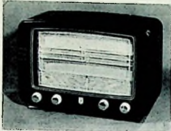
BX 321 A f 210,- afm. 27 x 40 x 18 cm drie golfgebieden 5 buizen met 8 functies
