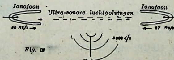
Demodulatie van twee staande ultra-sonore trillingen
