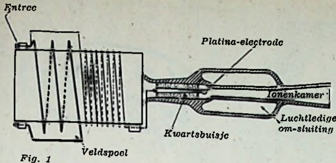
Fig. 1 Principe van de nieuwste „Ionofoon“
